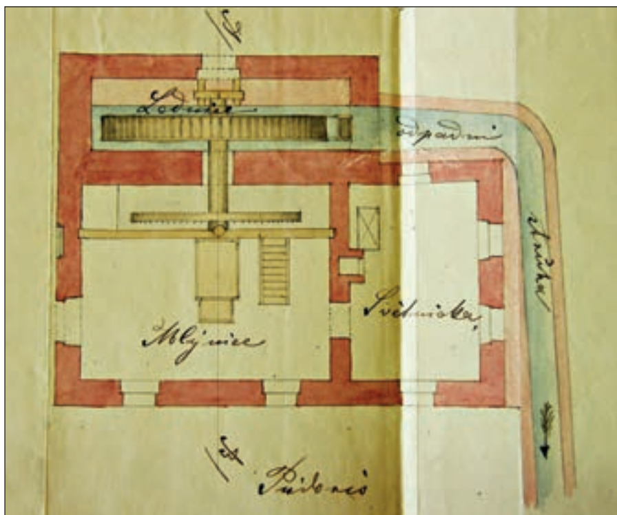
Půdorys mlýnice nerealizovaného Pičmanova mlýna na mletí pilin u čp. 51 (SOKA, 1875)
