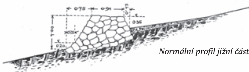
Profil valu v rozšíření v jižní části.
